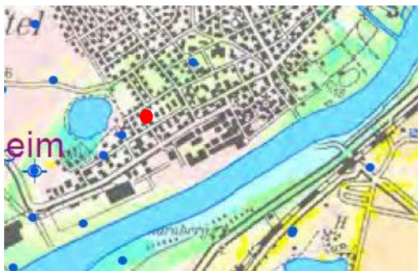
Abb. 17: Grundwasserflurabstand (Quelle: HLUG, 2015)
