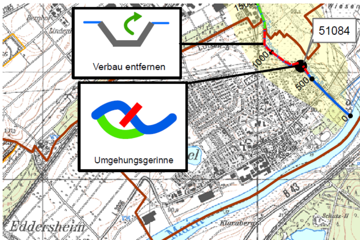
Abb. 40: Umsetzung Maßnahmenprogramm Schwarzbach, Potenzielle Maßnahmen - Durchgängigkeit und Morphologie (Ausschnitt Übersichtslageplan Sydro Consult, April 2012)
