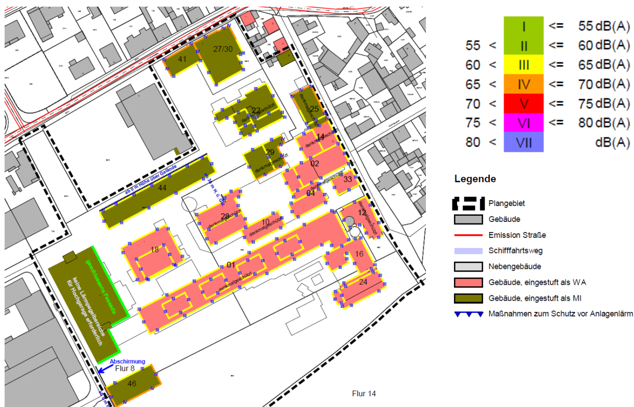
Abb. 36: Maßgebliche Außenlärmpegel nach DIN 4109-2 (Quelle: Schalltechn. Untersuchung Krebs+Kiefer Fritz AG, 2017)
