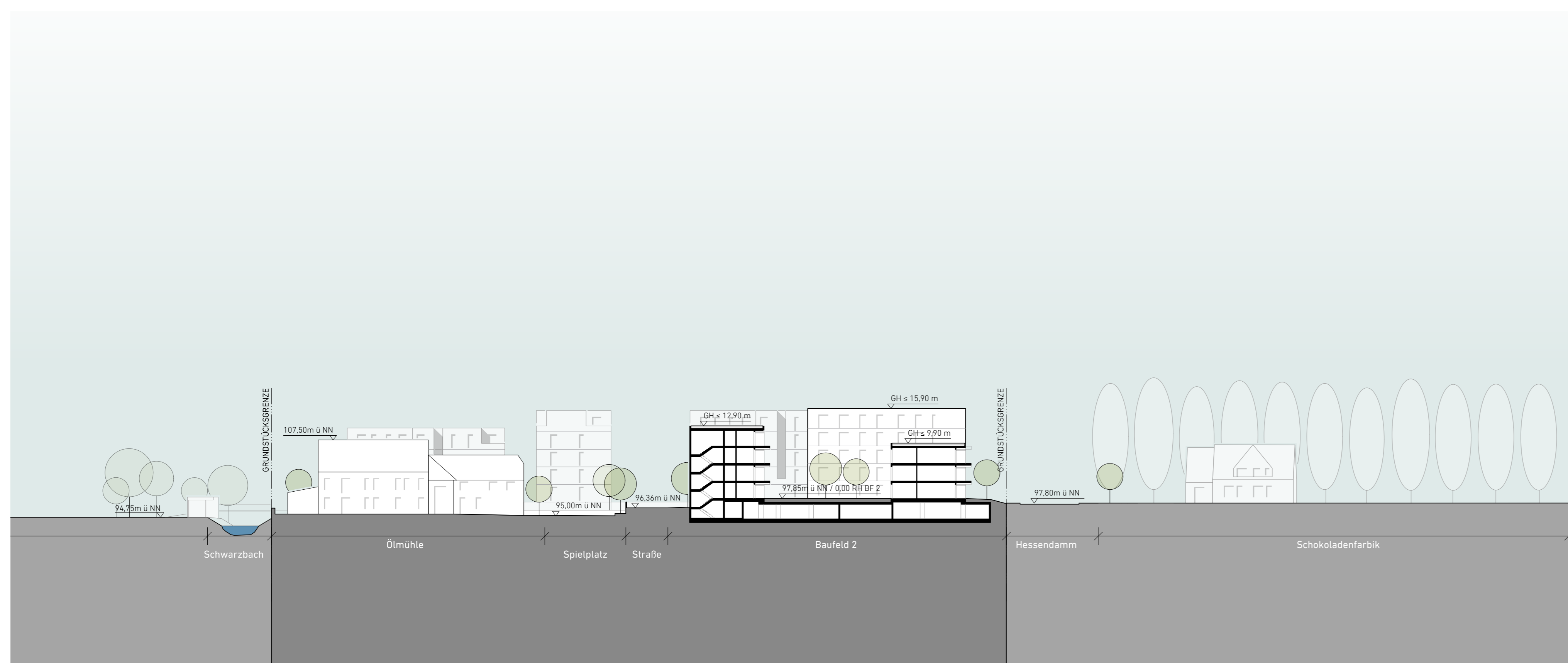
Prinzip-Schnitt B-B Ölmühle/ Baufeld 2 M 1:500
