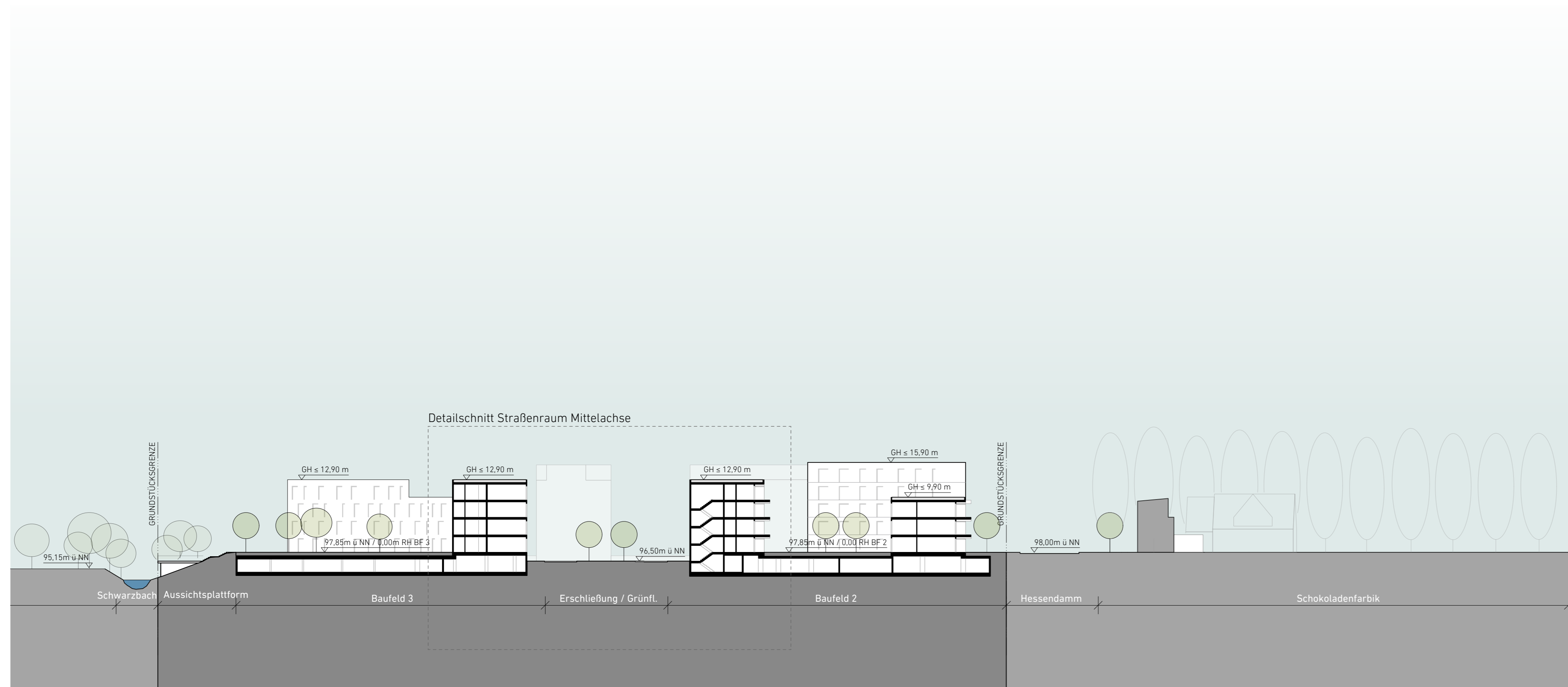
Prinzip-Schnitt A- A Baufeld 3 / Baufeld 2 M 1:500
