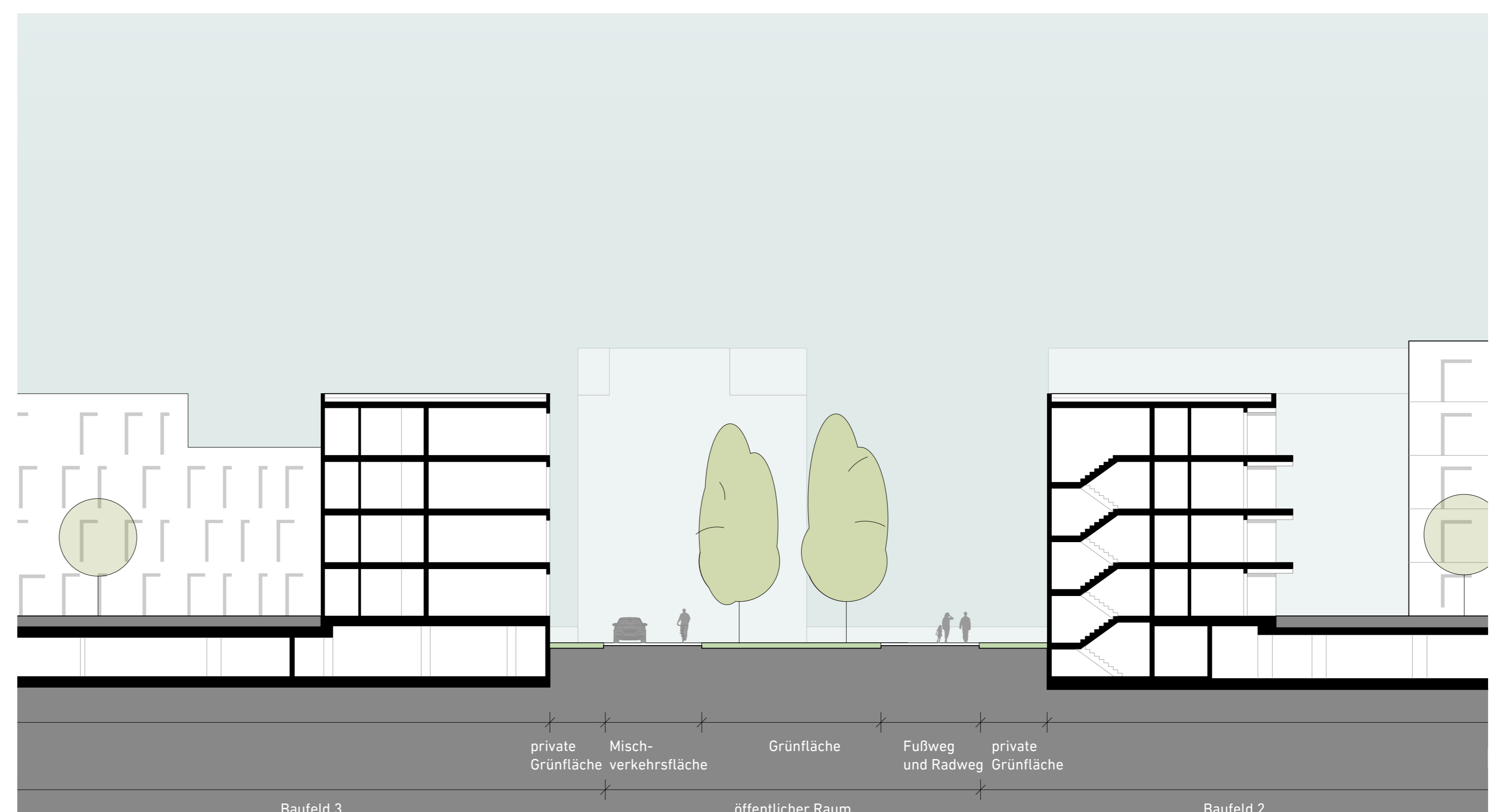
Detailschnitt D-D Straßenraum Mittelachse M 1:200
