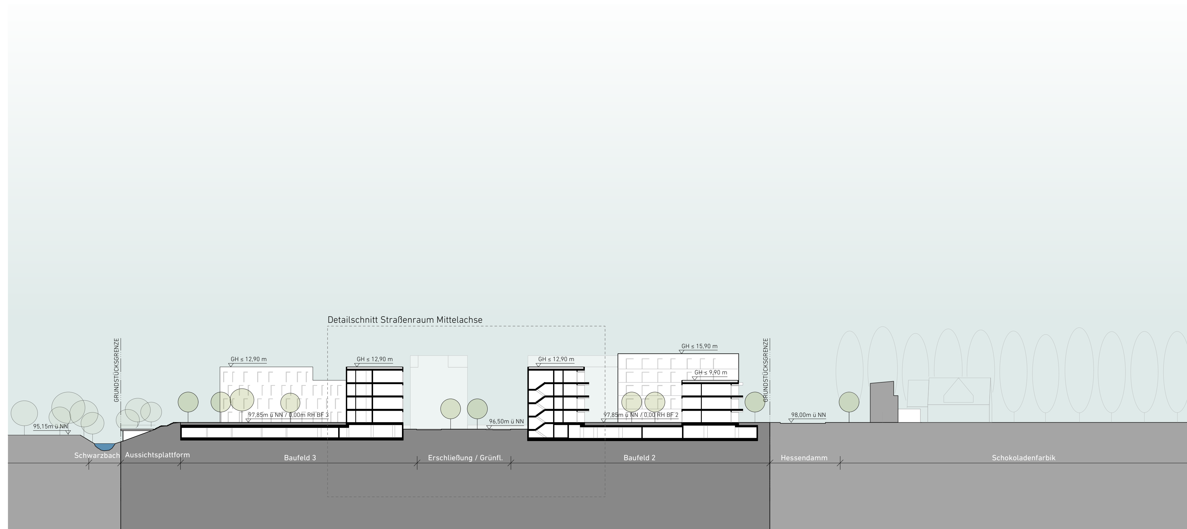
Prinzip-Schnitt A- A Baufeld 3 / Baufeld 2 M 1:500
